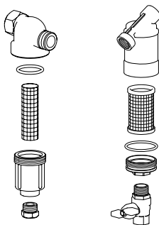
Filtros de Línea
